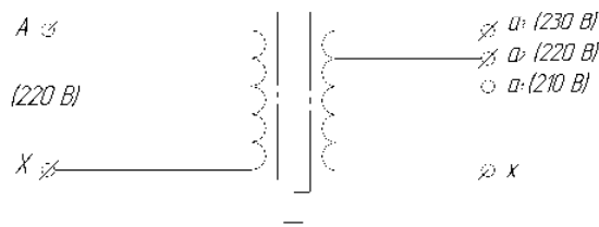
Рисунок А.2 Принципиальная электрическая схема трансформатора ОЛ-0,3/35
