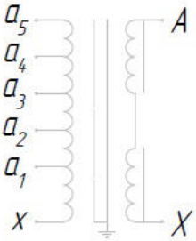
Рисунок А.6 – Принципиальная электрическая схема трансформаторов
