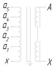
Рисунок А.8 – Принципиальная электрическая схема трансформаторов
