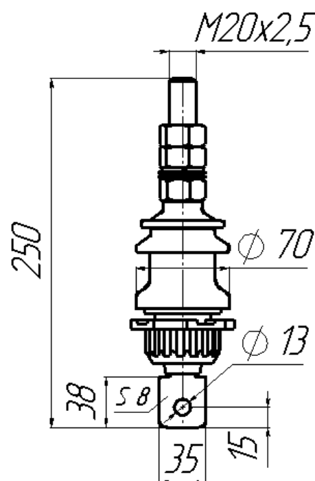
Рис. Б.6 – Вводы НН для трансформаторов
