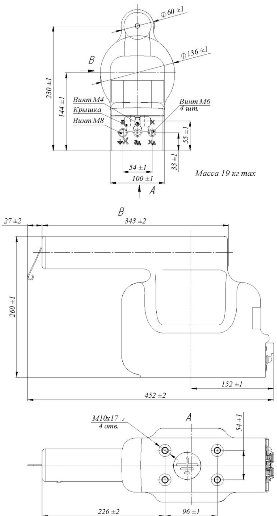
Рисунок Б.4 Внешний вид трансформаторов ЗНОЛ.01ПМИ
