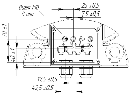
Рисунок А.2 Клемник для трансформаторов ЗНО/14-35 III (остальное см. рисунок А.1, крышка условно не показана)
