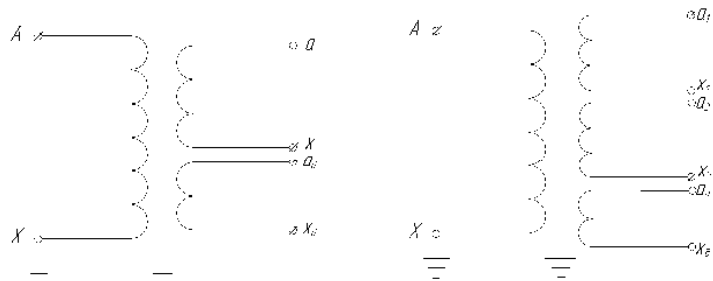
Рисунок А.3 Принципиальная электрическая схема трансформатора ЗНО/1-35(27) III
