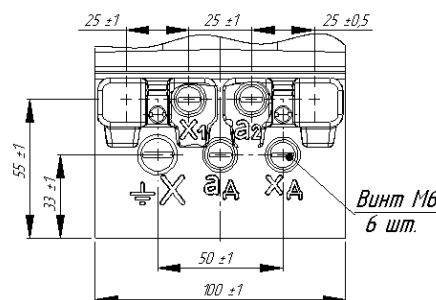
Рисунок А.5 Клеммник для исполнения ЗНОЛ.06.4 (остальное см. рисунок А.1)
