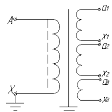
Рисунок А.3 Принципиальная электрическая схема для исполнений ЗНОЛ.06.4
