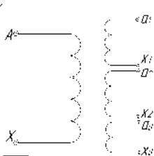
Рисунок Б.4 Принципиальная электрическая схема трансформатора ЗНОЛ.06.4-35
