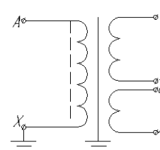
Рисунок А.2 Принципиальная электрическая схема трансформаторов ЗНОЛ.06
