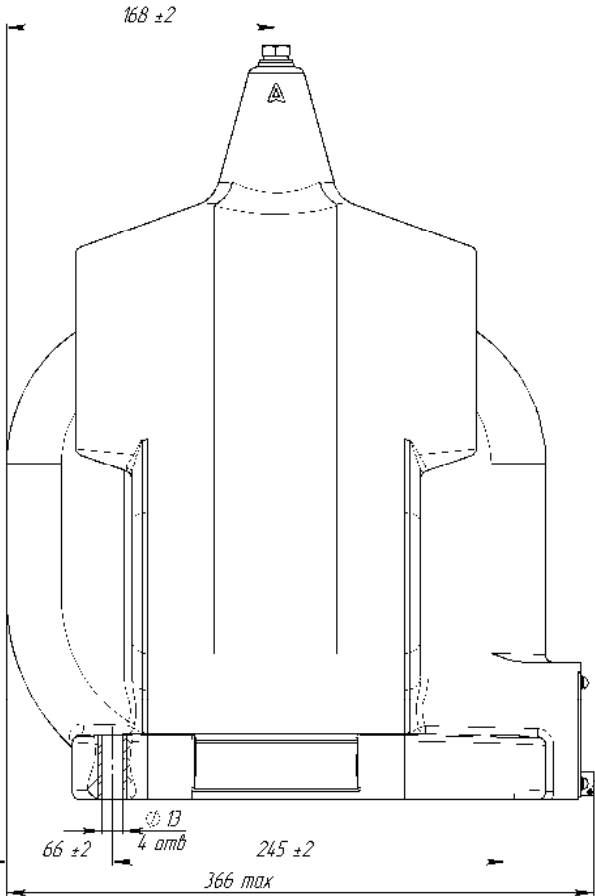
Рисунок Б.2 Клемник для исполнения ЗНОЛ.06.4-35 (остальное – см. рис. Б.1, крышка условно не показана)
